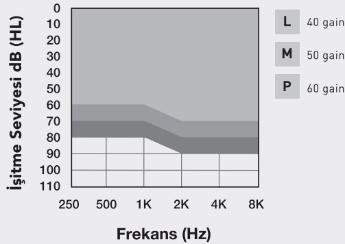
Standart Hoparlör ile RIC
